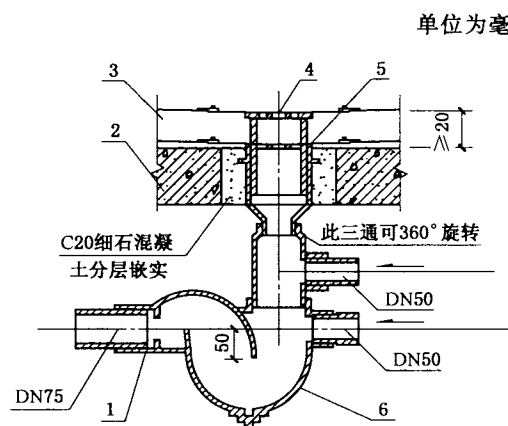
图 A.5 密闭式地漏
